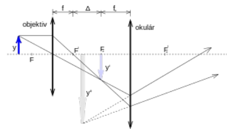
Znárodnění ohniskových vzdáleností a optického intervalu na schématu optického mikroskopu.
