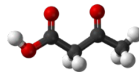
Kyselina acetoctová 3D
