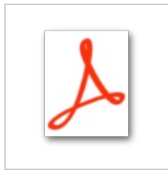
Radioaktivita.pdf 0 × 0; 1,27 MB
