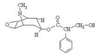
Skopolamin
