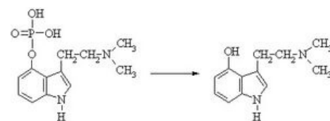
Psilocybin
