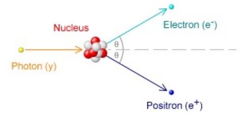
Tvorba elektron-pozitronového páru
