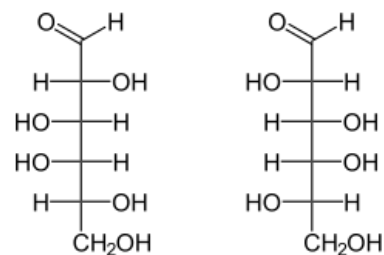
D-Galactose L-Galactose
