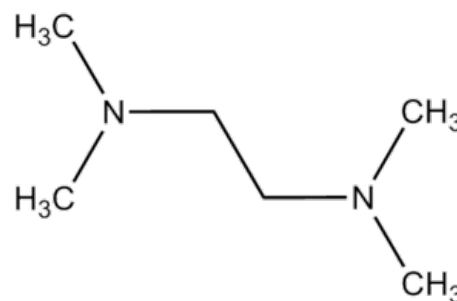
TEMED
