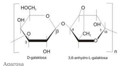
Agarosa
