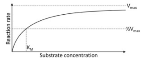
Graf kinetiky podle Michaelise a Mentenové
