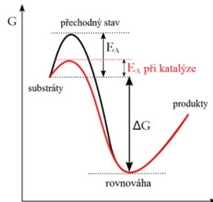
Aktivační energie
