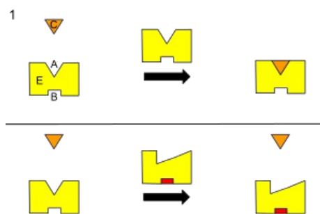
Vazba inhibitoru na molekulu enzymu: A - aktivní místo, B - allosterické místo, C - substrát, D - inhibitor, E - enzym
