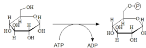
Fosforylace glukózy
