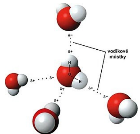
Vodíkové můstky podílejí se na vazbě mezi enzymem a substrátem
