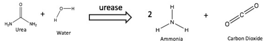
Ureáza katalyzující reakci - schéma
