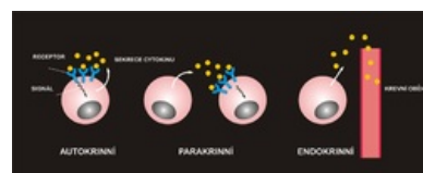
Působení cytokinů
