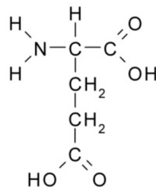
Kyselina glutamová
