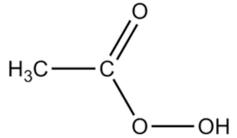
Kyselina peroxyoctová
