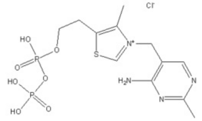
Thiamin pyrofosfát
