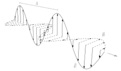
Elektromagnetická vlna
