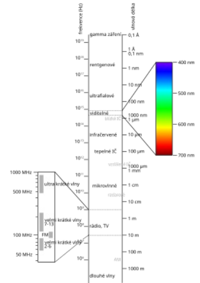
Elektromagnetické spektrum
