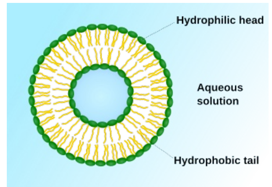
Schéma jednoduchého lipozomu
