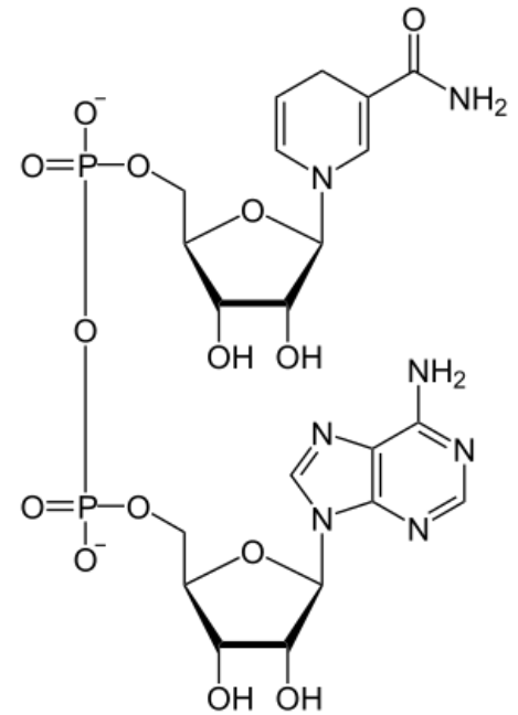
Struktura NADH
