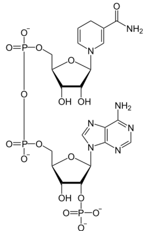
Struktura NADPH
